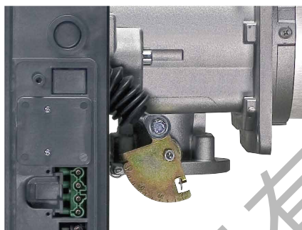
RS 34-44 MZ 系列燃烧器可变线凸轮示例。
